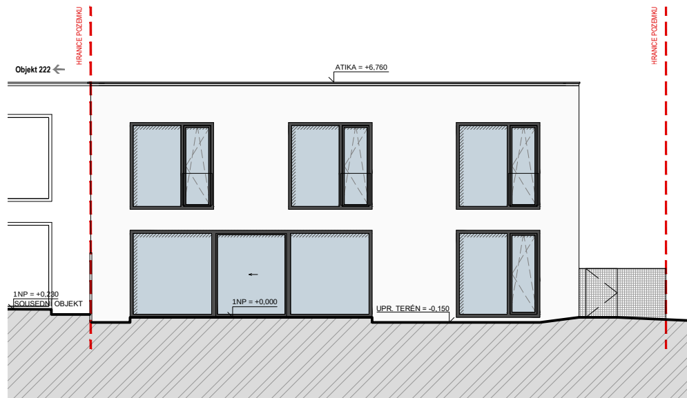
POHLED JIŽNÍ
