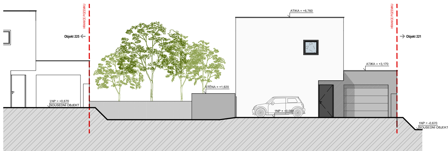
POHLED VÝCHODNÍ
