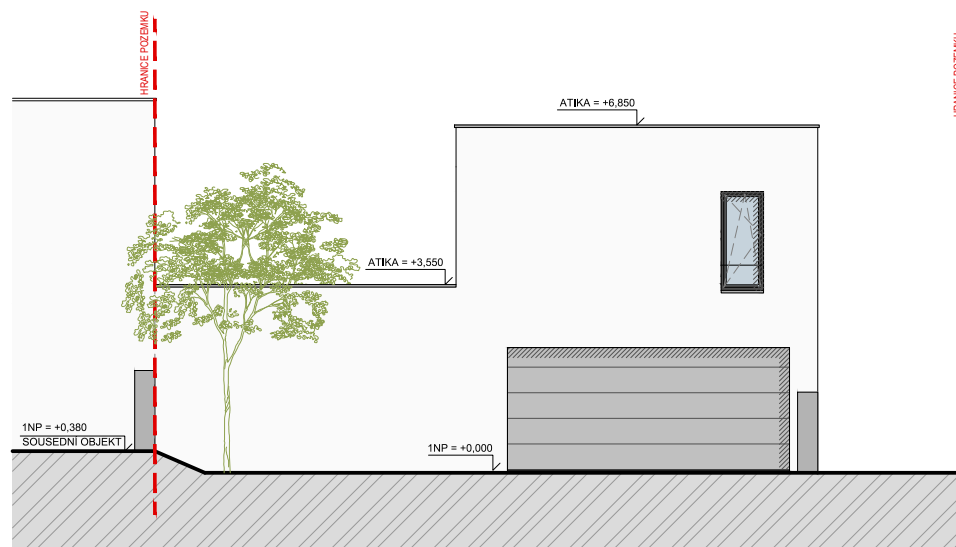
POHLED VÝCHODNÍ
