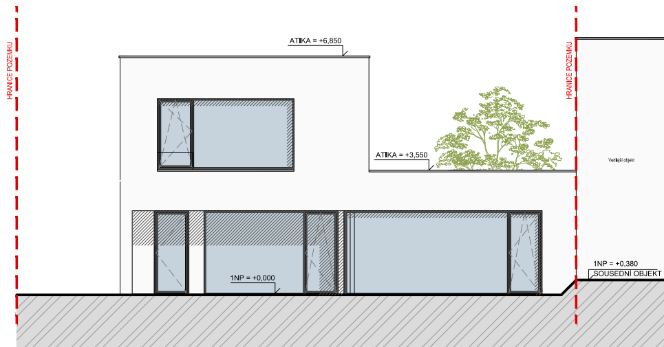
POHLED ZÁPADNÍ
